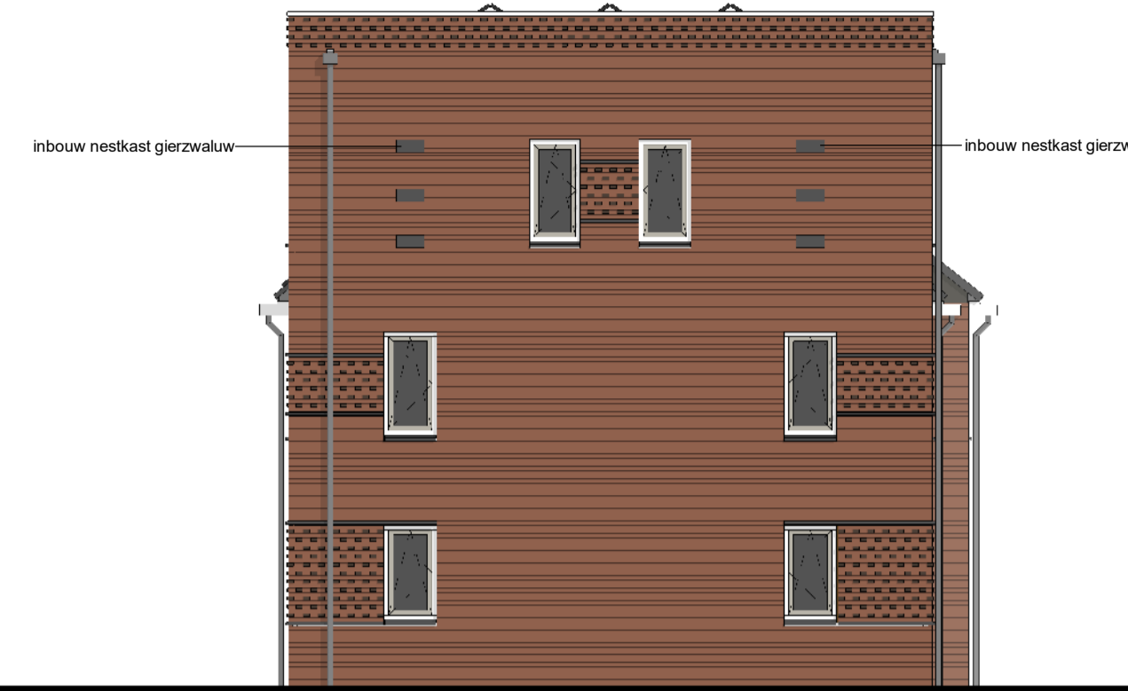
Rechter zijgevel 1 : 100
