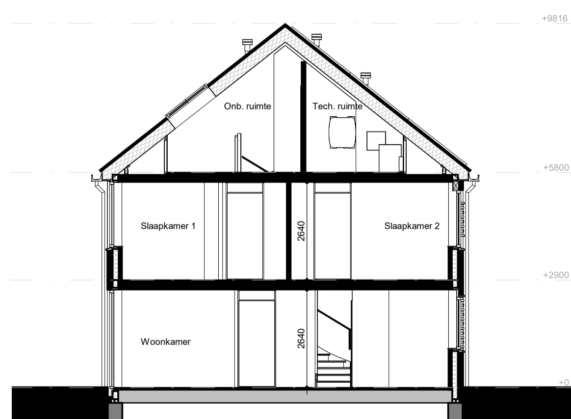
Doorsnede hoekwoning 1 : 100
