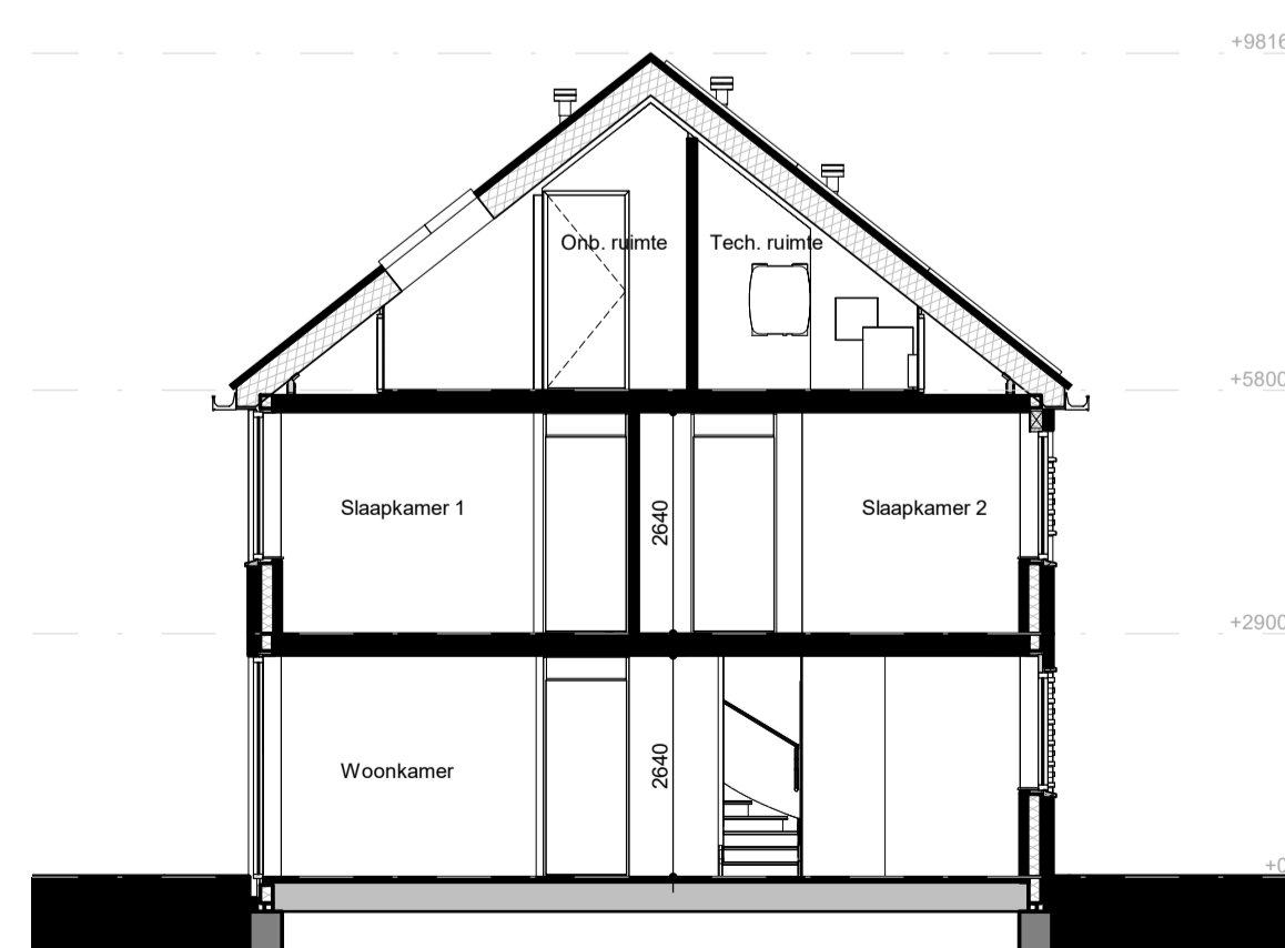
Doorsnede tussenwoning 1 : 100
