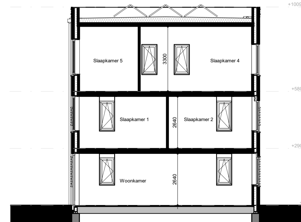
Doorsnede hoekwoning, plat dak 1 : 100
