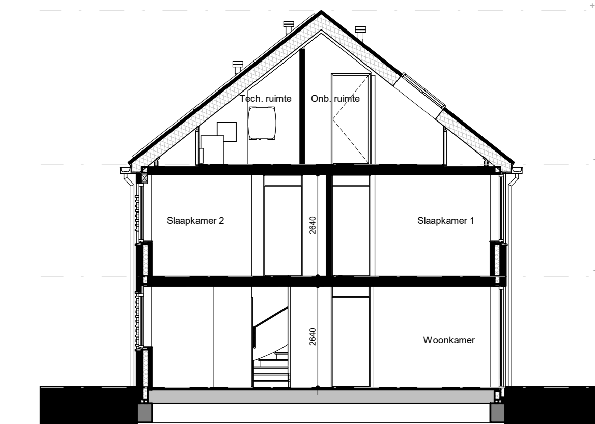
Doorsnede tussenwoning 1 : 100
