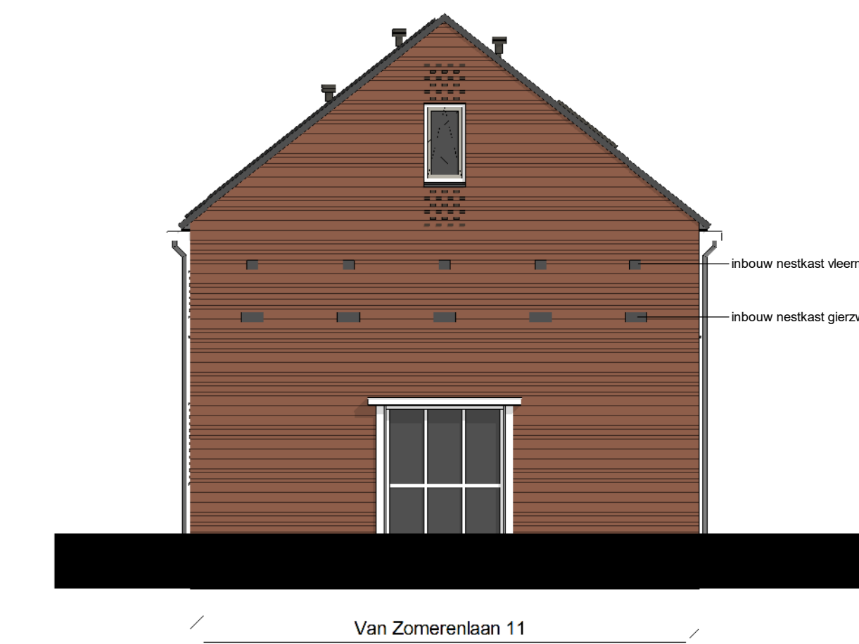
Rechter zijgevel 1 : 100
