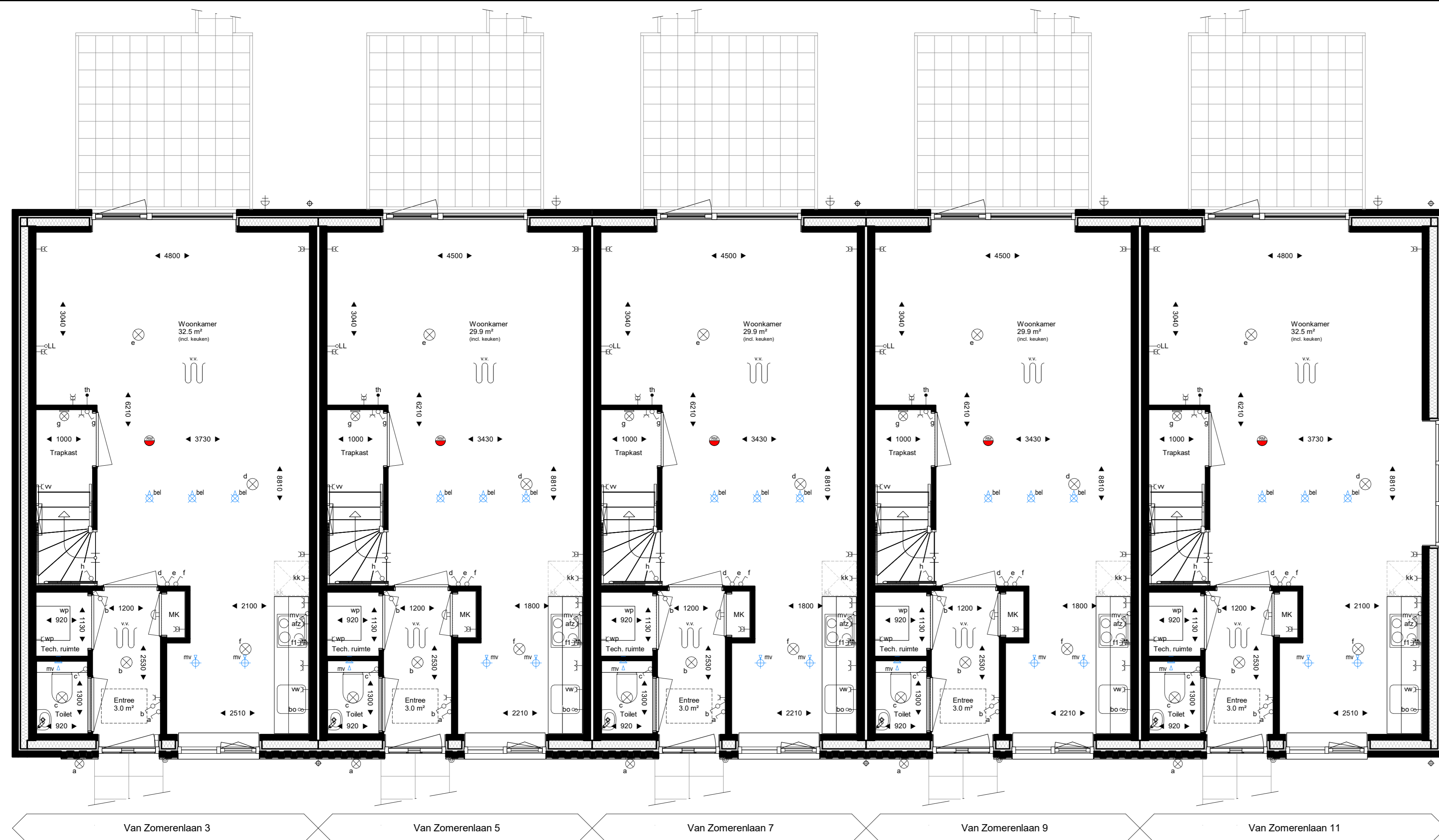
Begane grond 1 : 50
