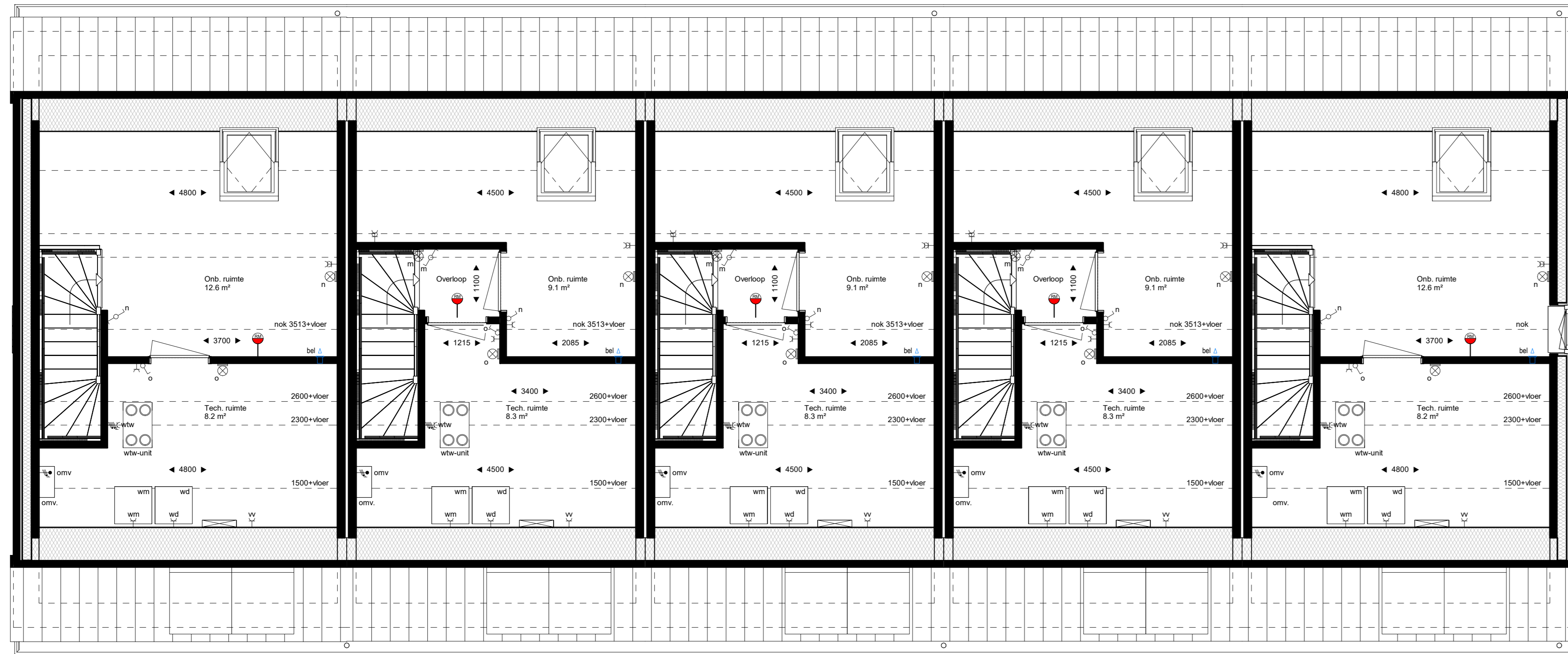
Eerste verdieping 1 : 50
