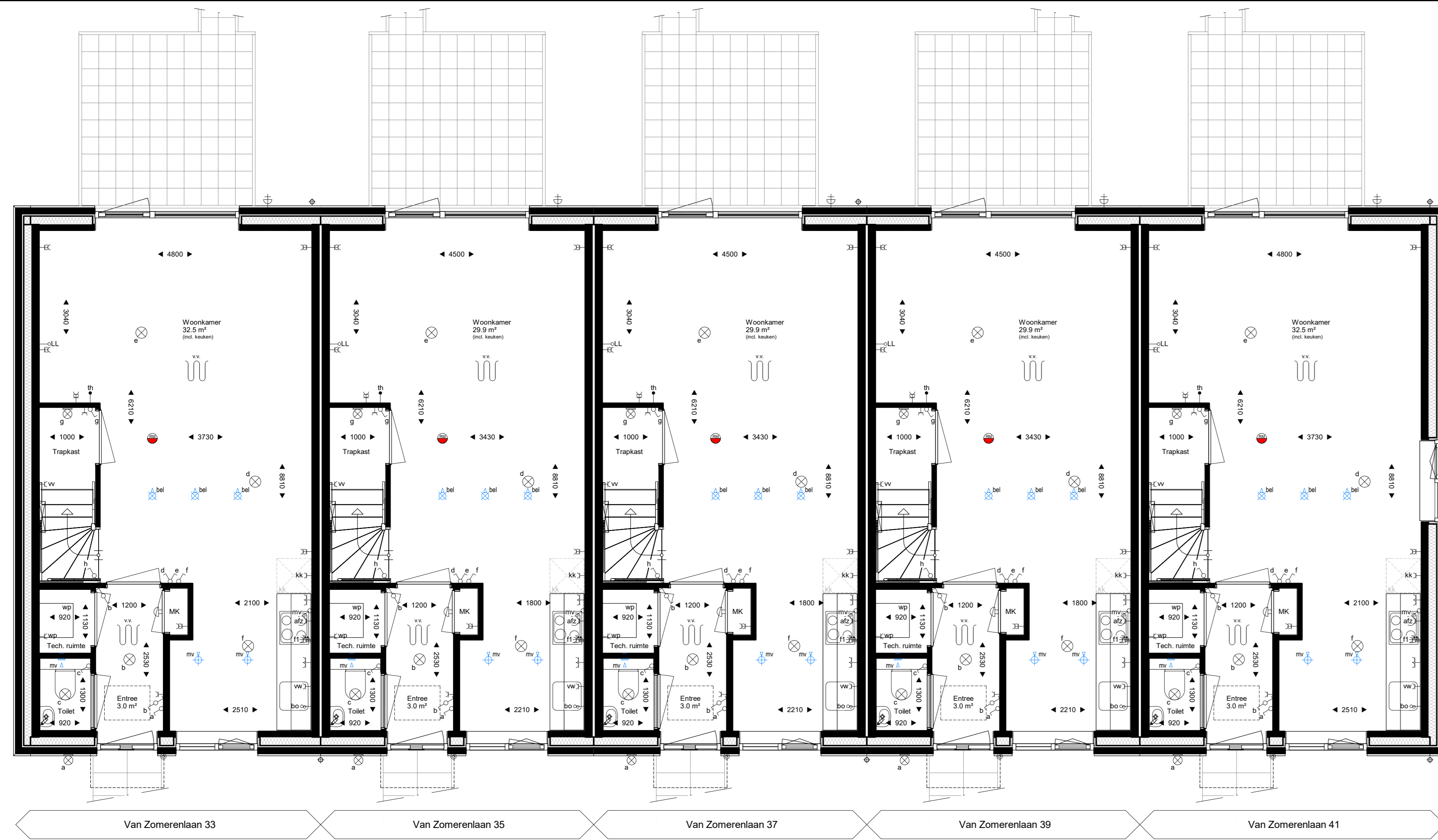
Begane grond 1 : 50
