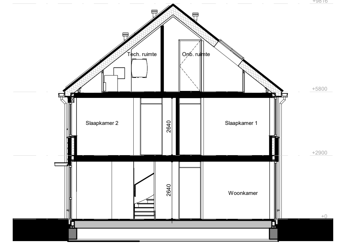
Doorsnede tussenwoning 1 : 100
