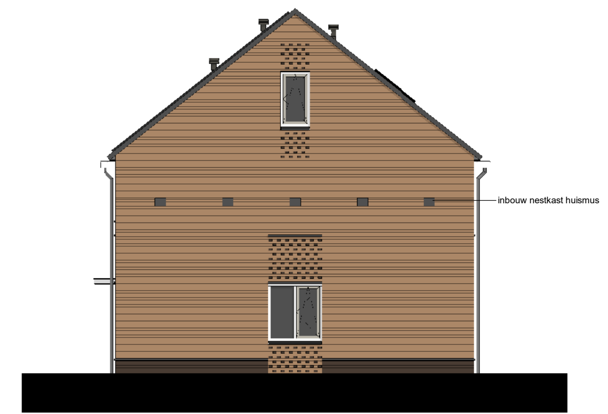
Rechter zijgevel 1 : 100
