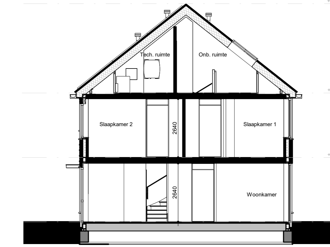
Doorsnede hoekwoning 1 : 100
