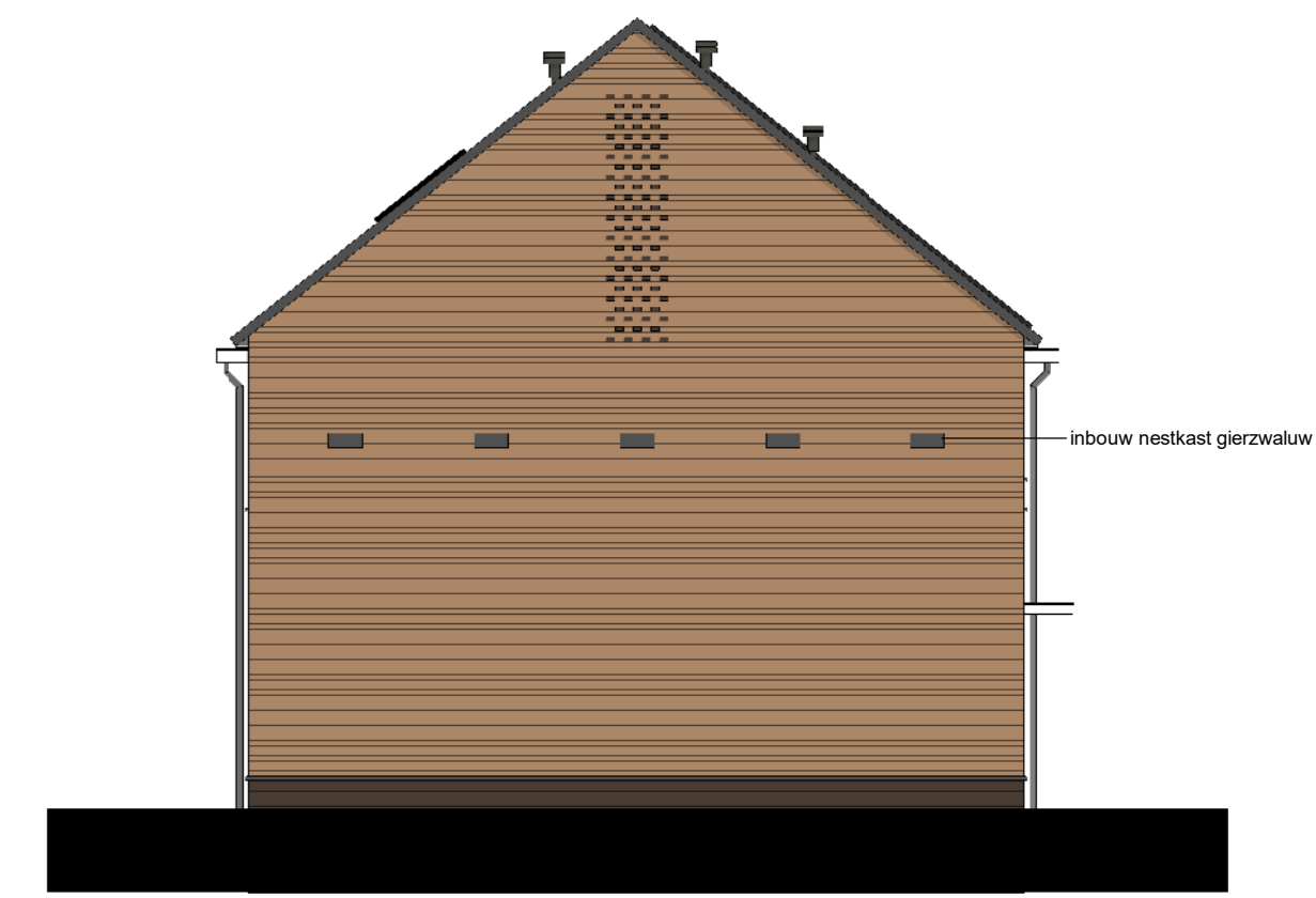
Linker zijgevel 1 : 100
