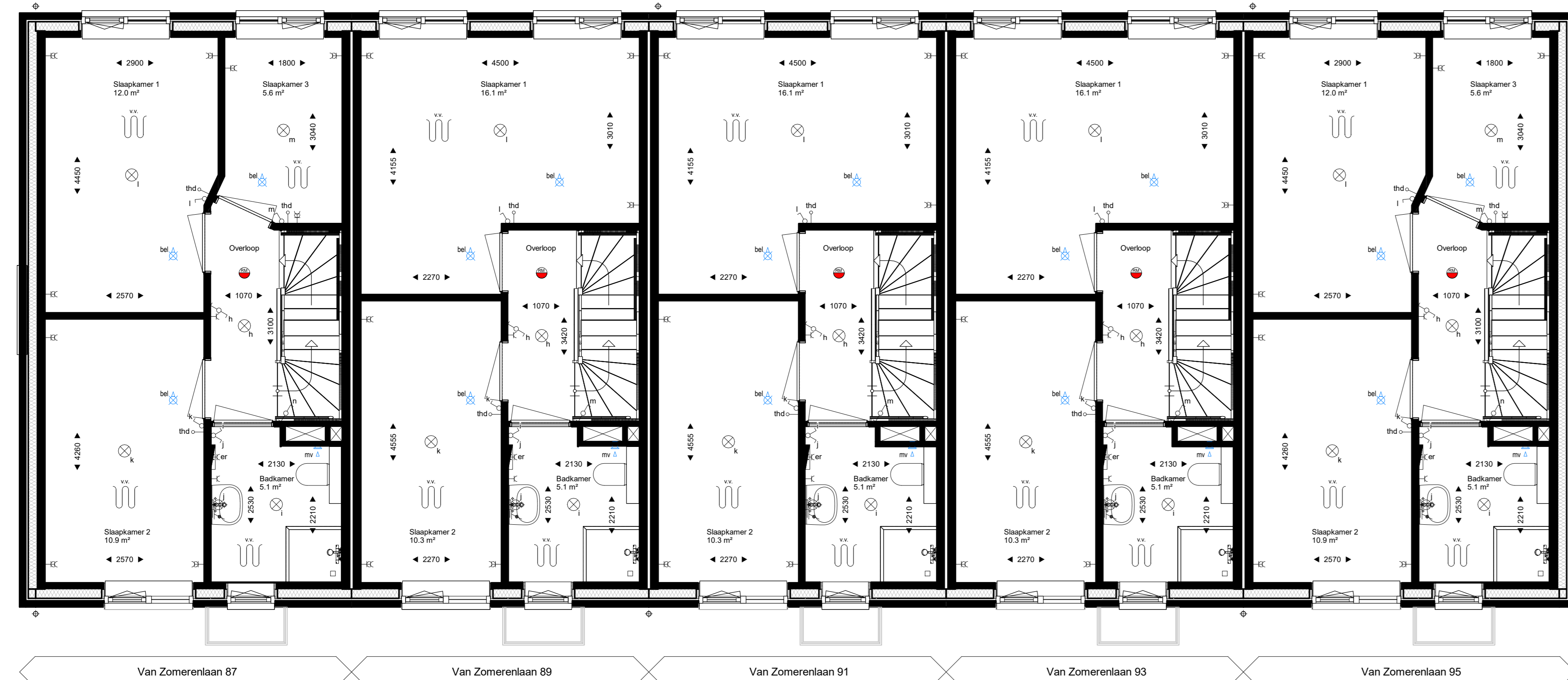
Eerste verdieping 1 : 50
