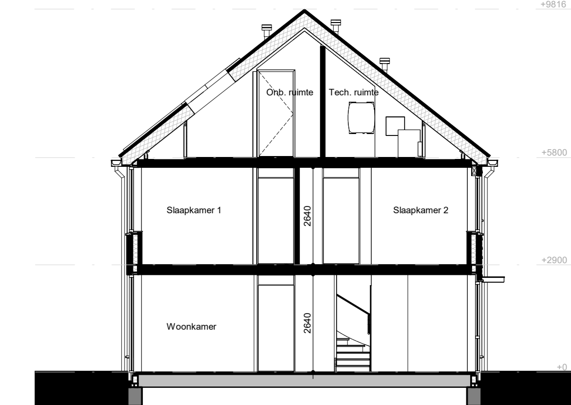
Doorsnede tussenwoning 1 : 100
