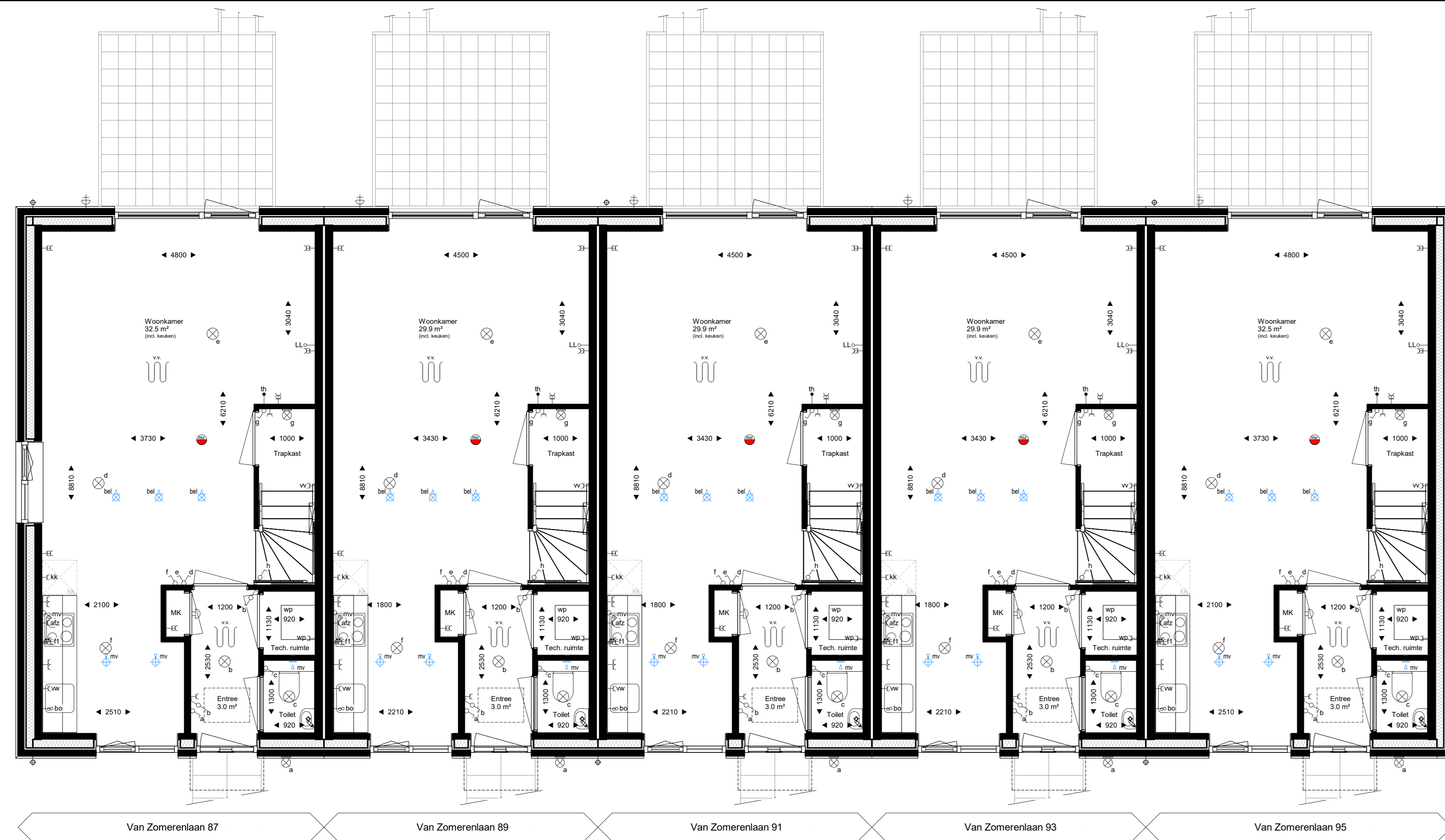
Begane grond 1 : 50
