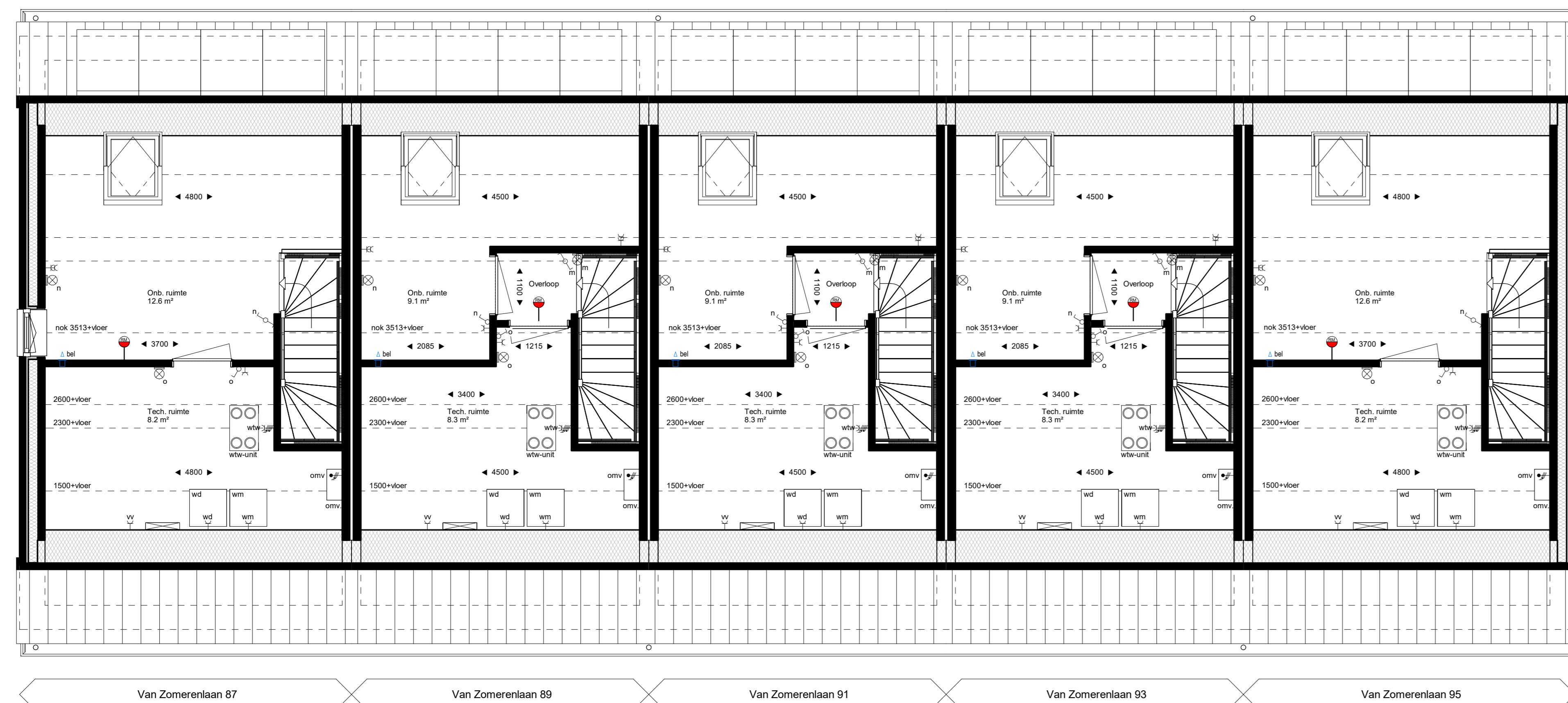
Tweede verdieping 1 : 50
