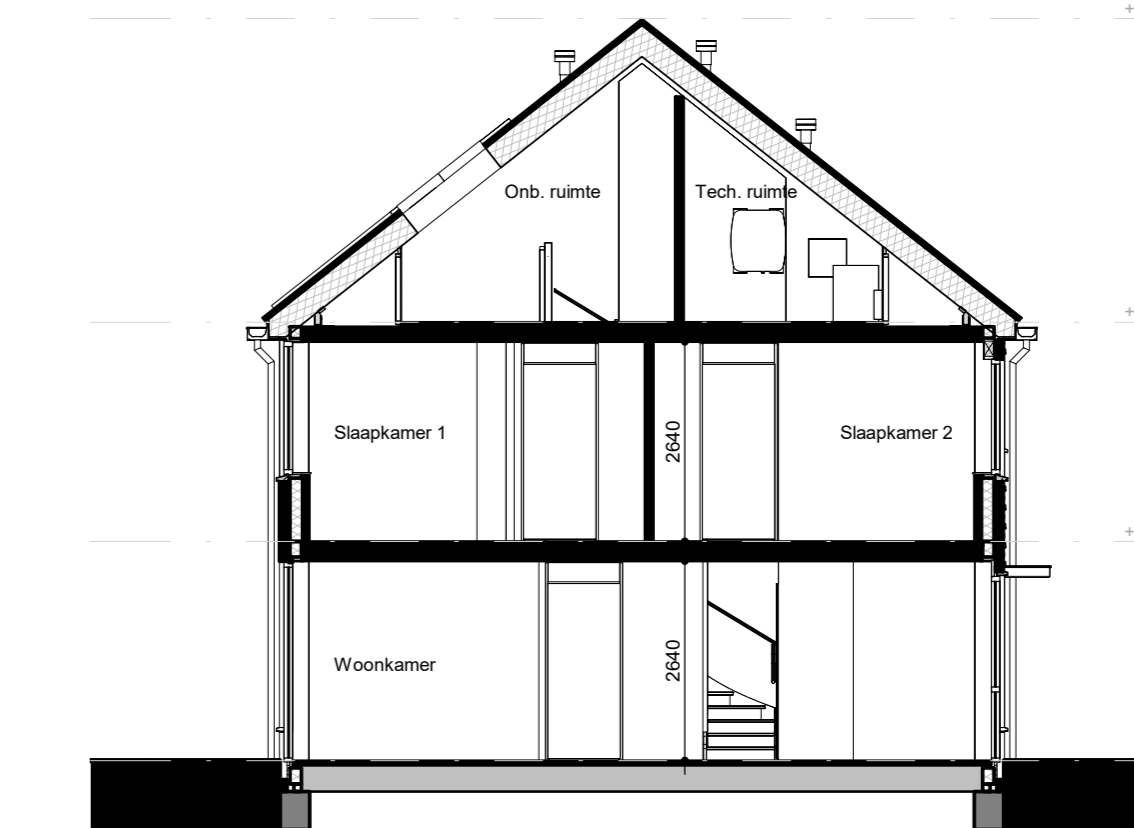
Doorsnede hoekwoning 1 : 100
